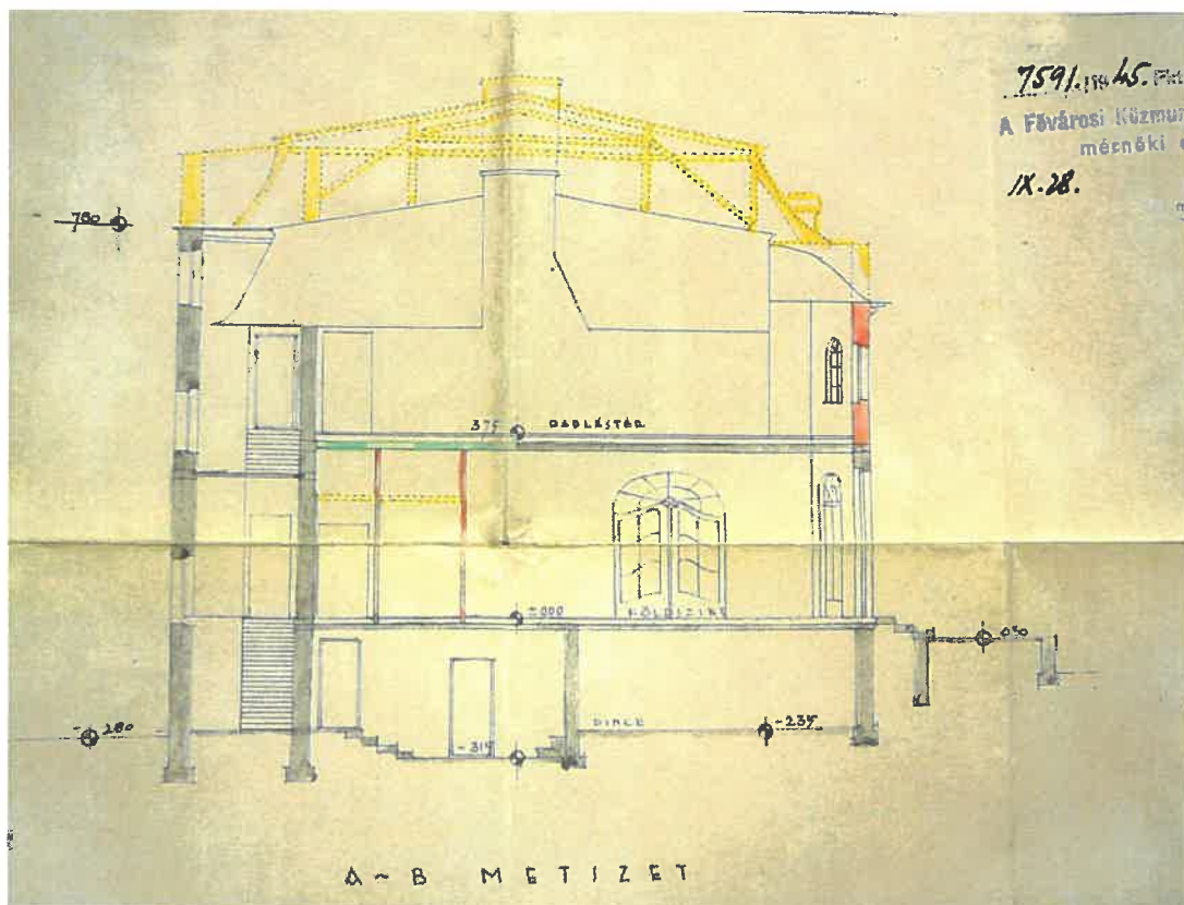
A padlástér átalakítási terve (a terasz nem megvalósult felszámolásával) és a metszet
