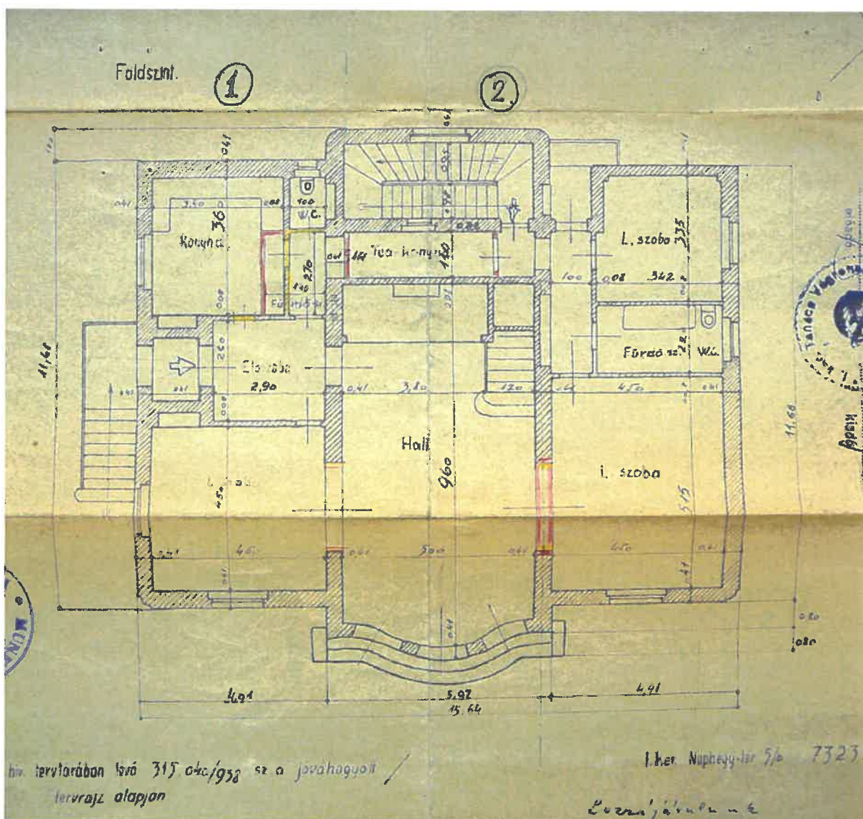
A földszint alaprajza (az 1945. évi helyreállítási terven még megvoltak a belépő fogadóter elegáns, ívelt, mélyített falfülkái)
