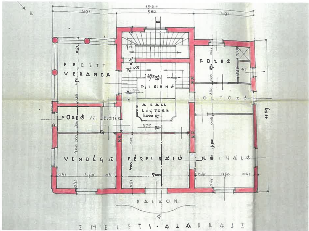
Az emelet alaprajza és a metszet
