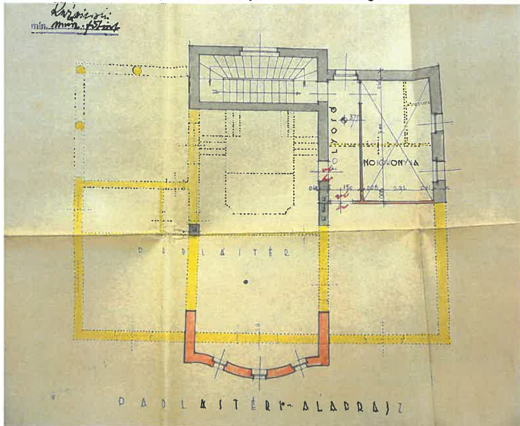
A padlástér átalakítási terve (a terasz nem megvalósult felszámolásával) és a metszet
