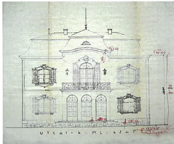
1938. az eredeti, megvalósult homlokzatterv
