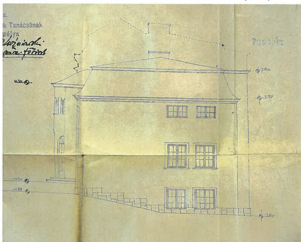
Az oldalhomlokzatok átalakítási tervei (az eredeti tetőidom kontúrjának jelzésével)
