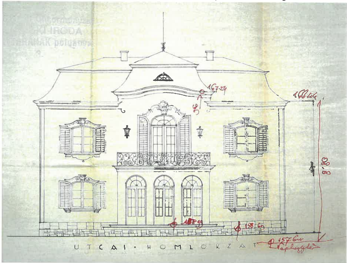
Az utcai (délkeleti) és a hátsókerti (északnyugati) homlokzatok
