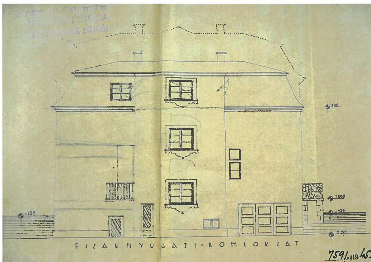
Az utcai és a hátsókerti átalakított homlokzat (az eredeti tetőidom kontúrjának jelzésével)
