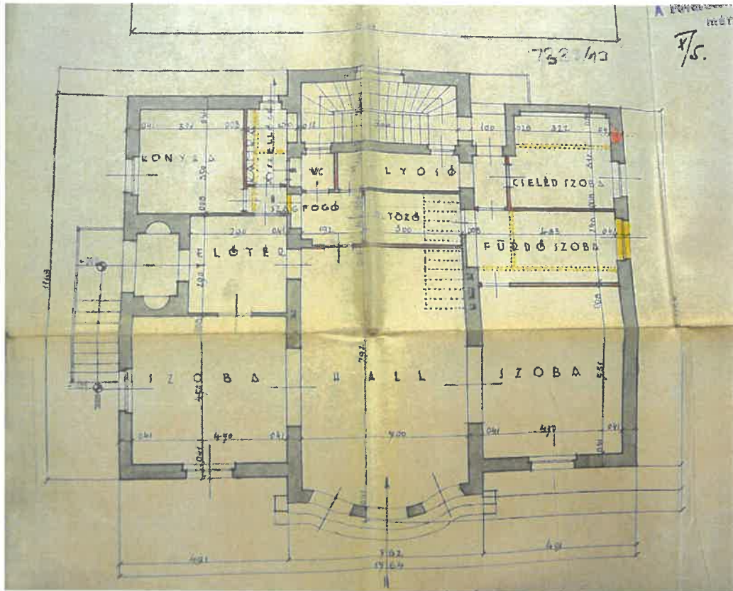
A földszint és a pince átalakítási terve
