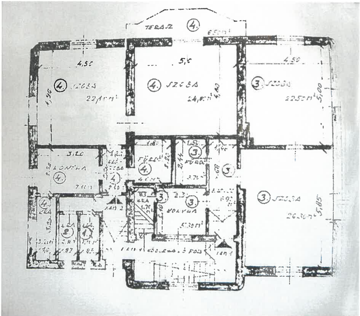
A részben a tetőtérbe rejtett, alacsony emelet kiépítése
