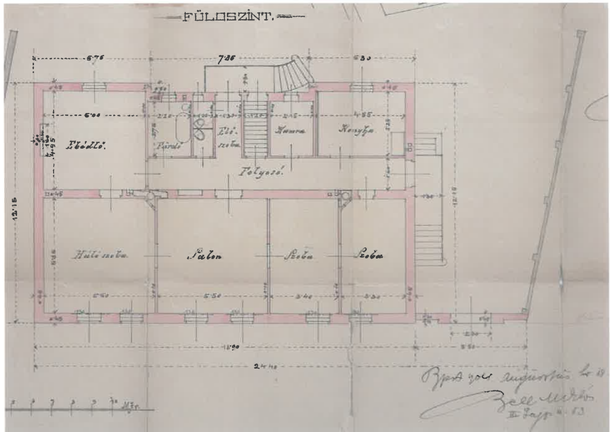
földszint alaprajza
