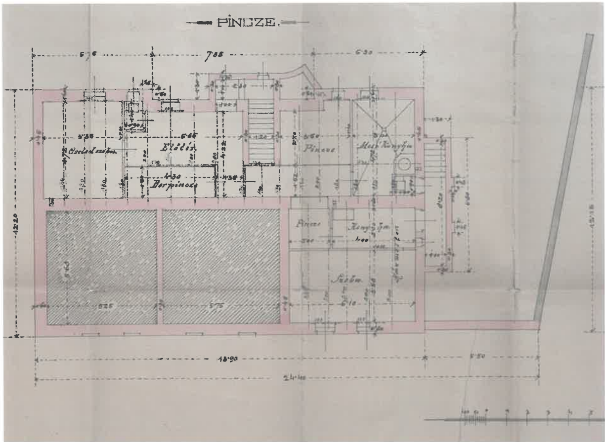
pince alaprajza
