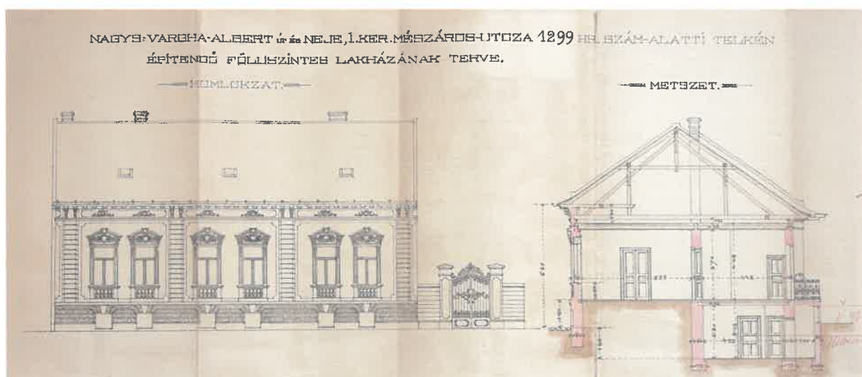
utcai homlokzat, metszet
