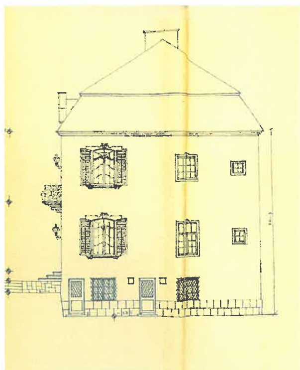
A hátsó- és az oldalhomlokzatok tervei
