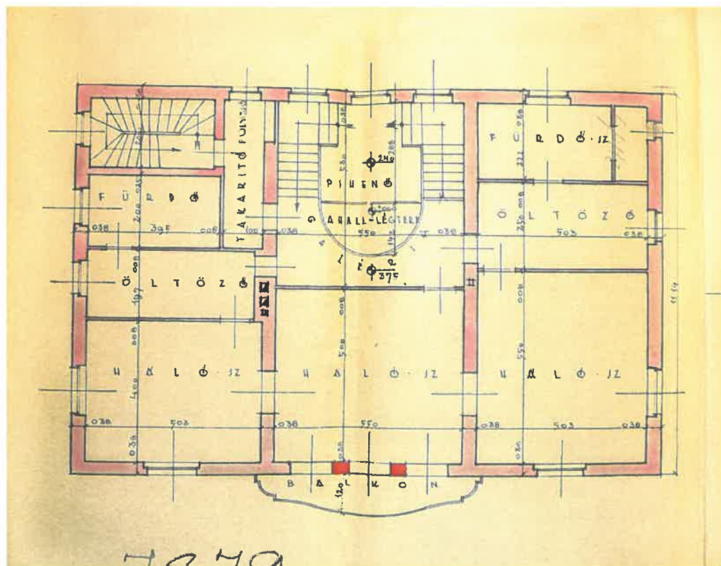
A villa földszinti és emeleti alaprajza
