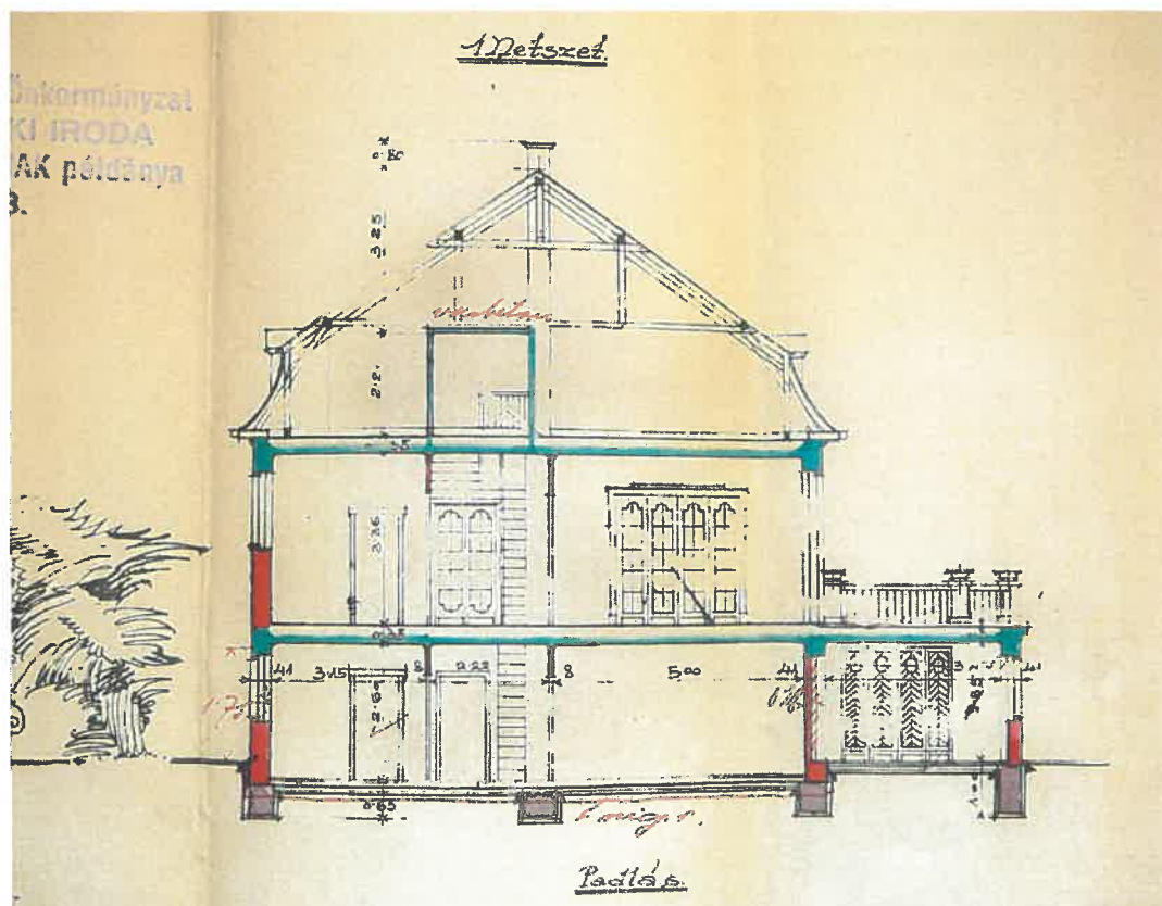
A tetőtér alaprajza és a ház metszete
