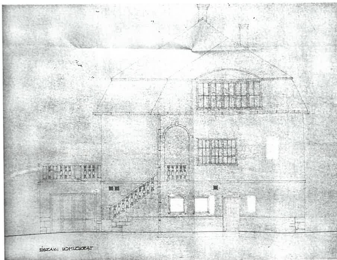
Az északi homlokzat terve
