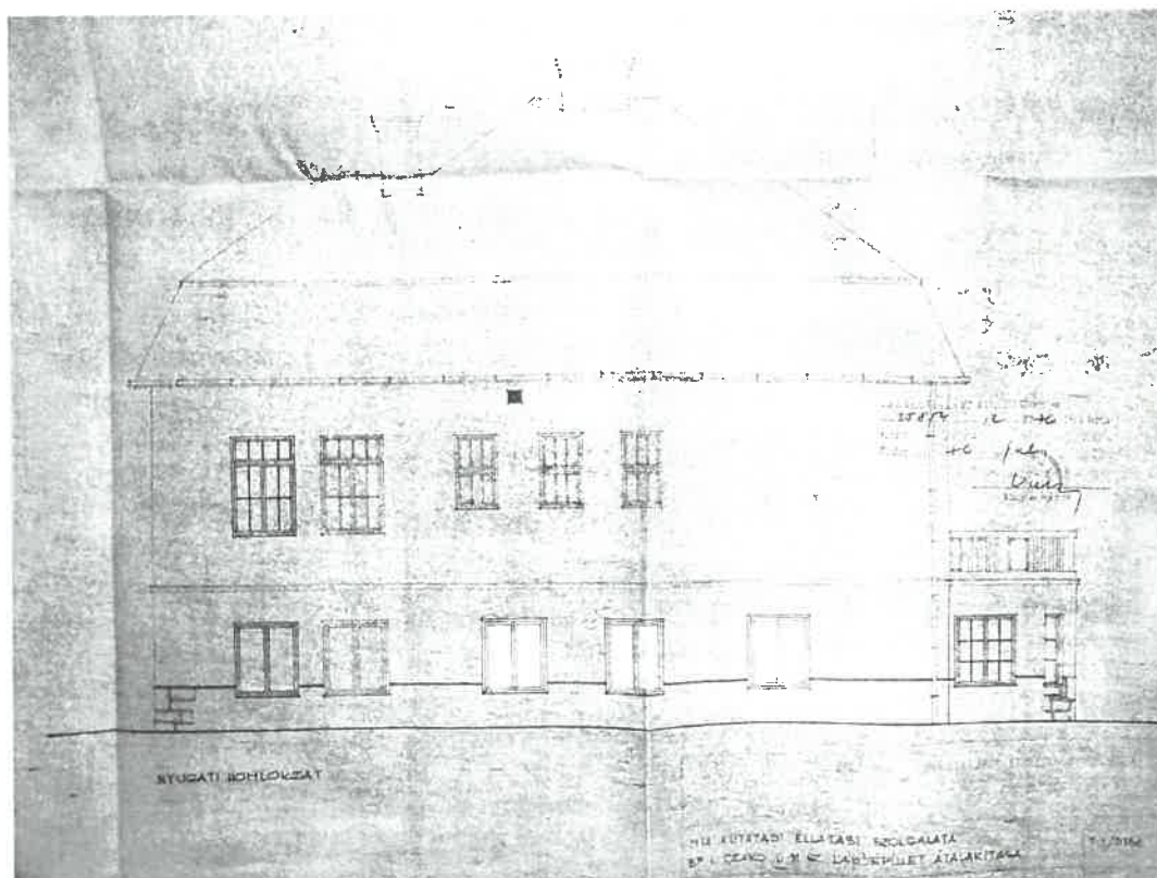
A nyugati homlokzat terve
