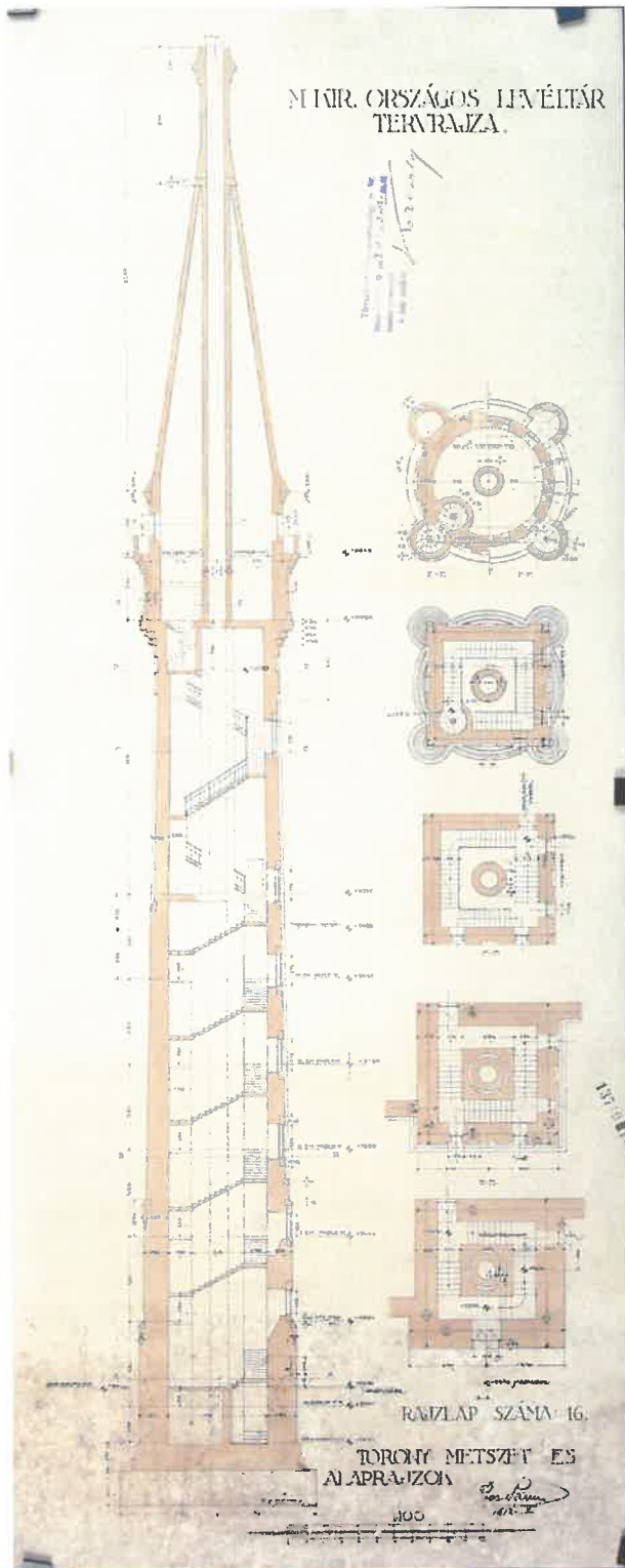
a torony metszete és alaprajza
