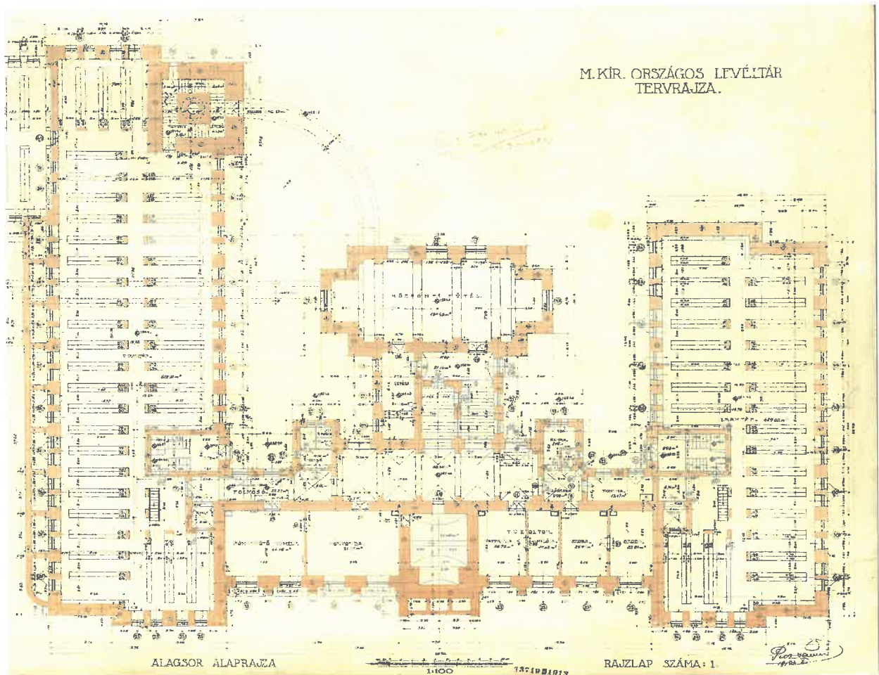
alagsor alaprajza, 1912
